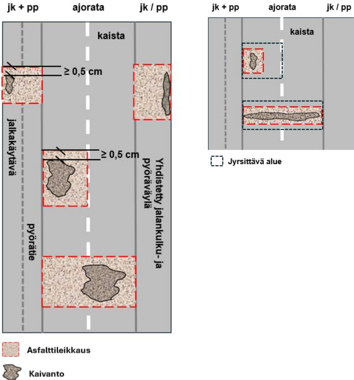
Kuva 2. Vanhan asfaltin leikkaustyöt ja uuden asfaltin päällystystyöt tehdään kuvien mukaisesti. Ajojänteillä, joilla on kaksi tai useampia sidottua kerrosta, kulutuskerros jyrsitään kuvan mukaisesti.
