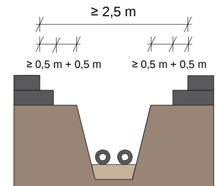
Asfaltin leikkausetäisyys reunan yli, useampi kerros asfalttia
