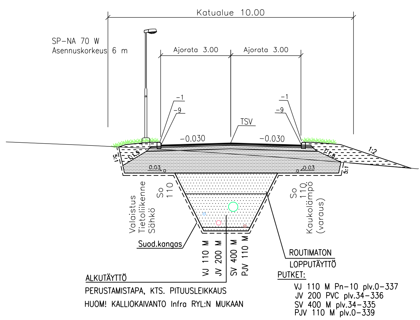
TYYPPIPOIKKILEIKKAUS 1:100 Palojoenkierto, eteläinen osa (pl 10)
