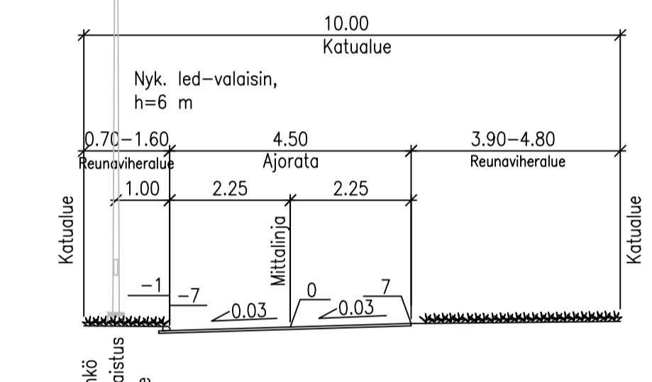
KOPPELONKUJA TYYPPIPOIKKILEIKKAUS, AJORATA
