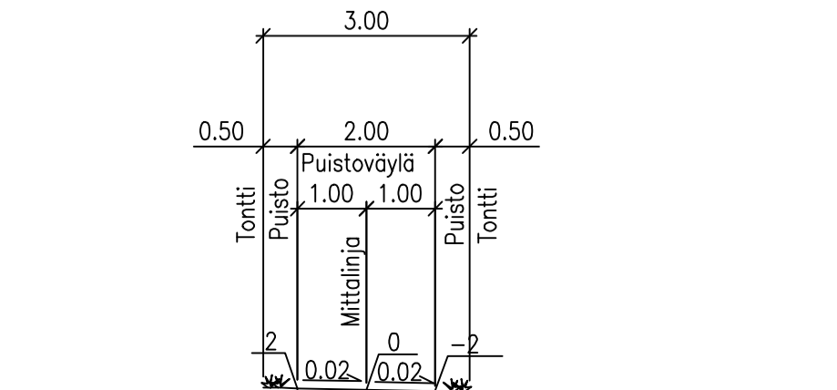
PUUSTOVÄYLÄT TYYPPIPOIKKILEIKKAUS
