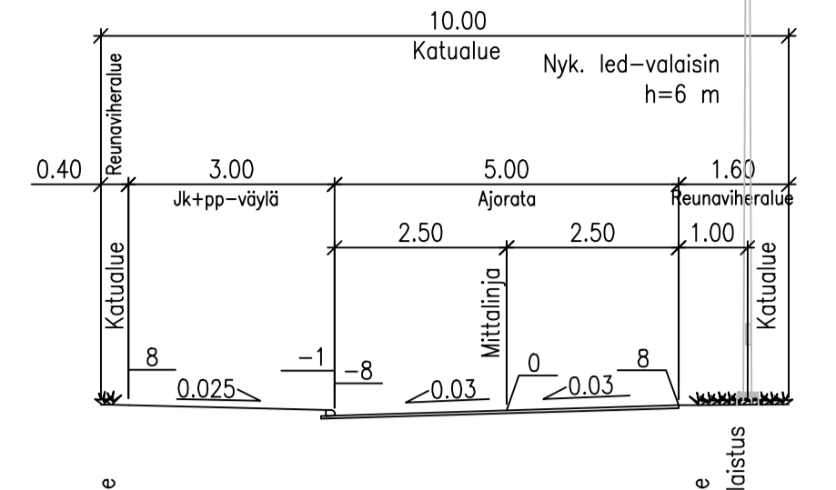
PALOKÄRJENKUJA B TYYPPIPOIKKILEIKKAUS, AJORATA
