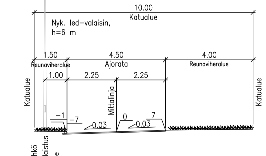
METSONKUJA PLV 45-200 TYYPPIPOIKKILEIKKAUS, AJORATA
