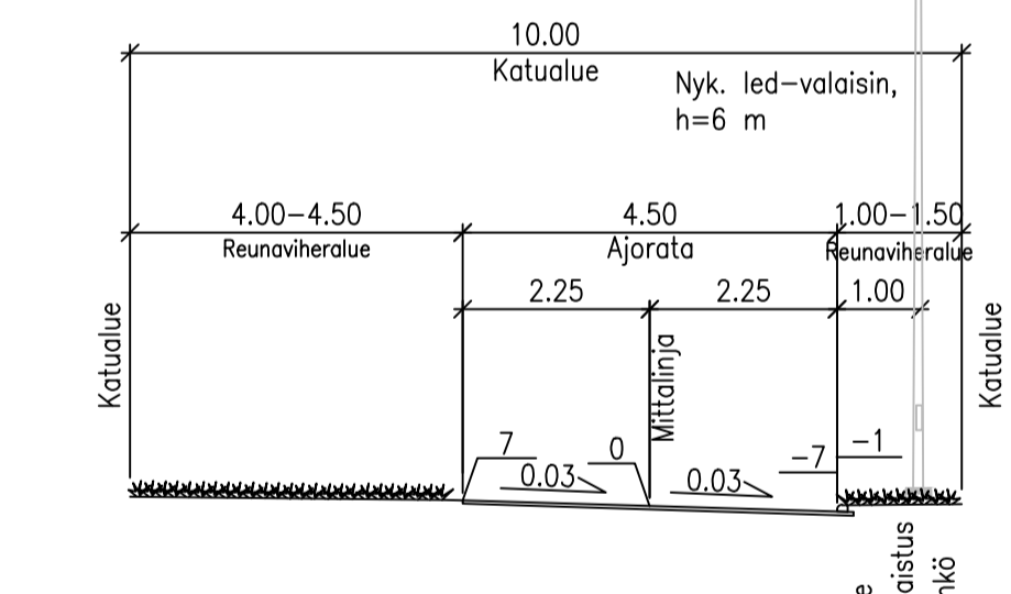
METSONKUJA PLV 0-45 JA PYYKKUJA TYYPPIPOIKKILEIKKAUS, AJORATA
