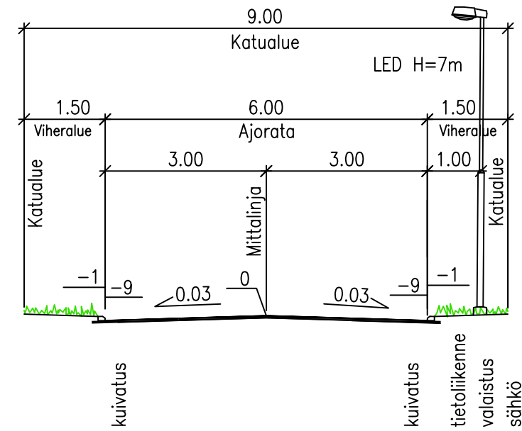
KOTIKATU TYYPPIPOIKKILEIKKAUS (PL 90)
