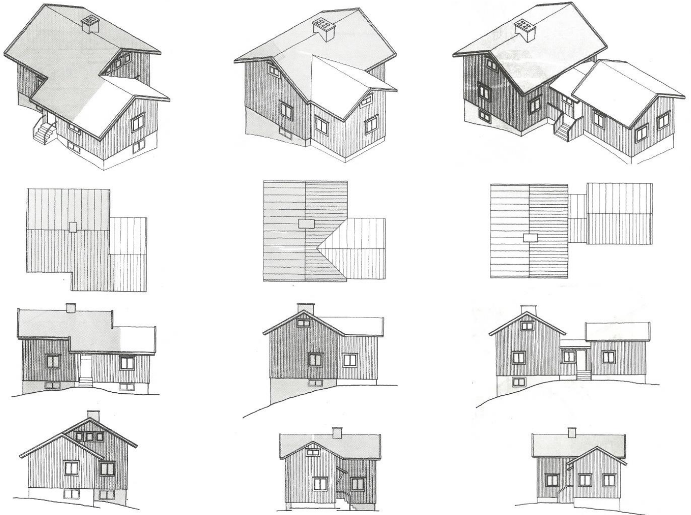
Kuva: Esimerkkejä rintamamiestalotyypisiin pientaloihin sopivista laajennuksista. (Cifuentes 1979, 50-51; 62-63; 69)
